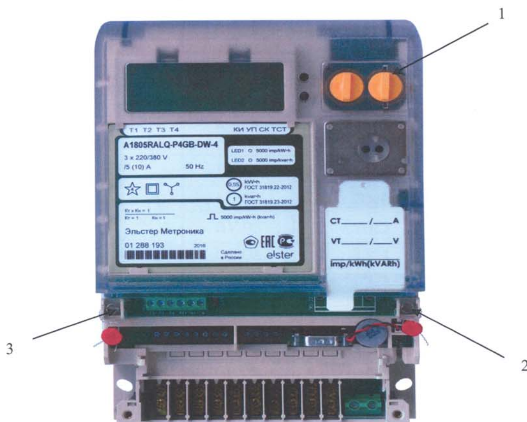
1 - пломба кнопки СБРОС; 2 - пломба поверителя; 3 - пломба ОТК завода-изготовителя Рисунок 1
